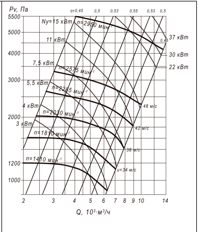
Аэродинамическая характеристика вентилятора ВЦП 7-40 №5
