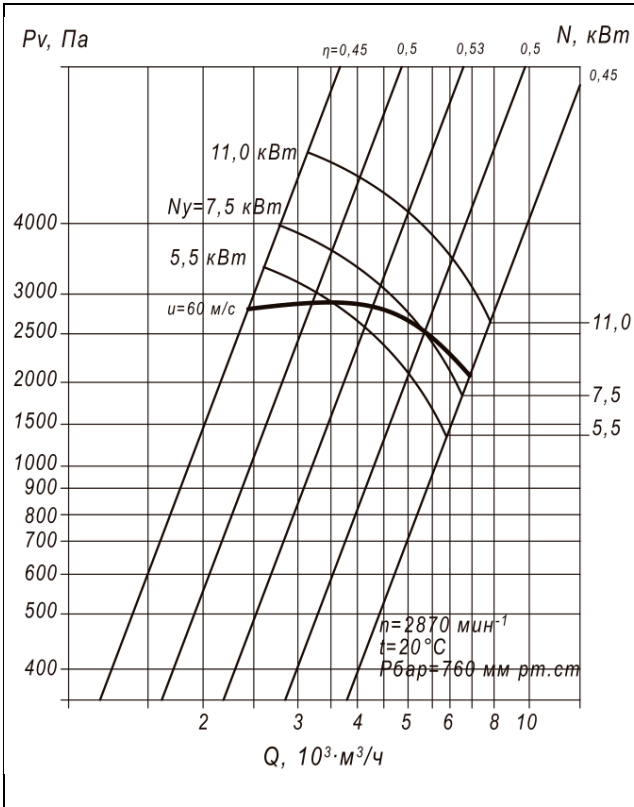
Аэродинамическая характеристика вентилятора ВЦП 7-40 №4
