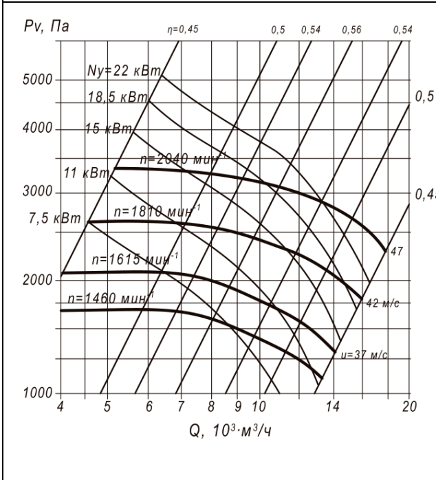
Аэродинамическая характеристика вентилятора ВЦП 7-40 №6,3
