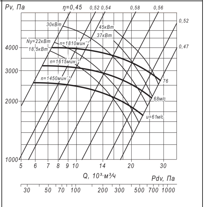
Аэродинамическая характеристика вентилятора ВЦП 7-40 №8
