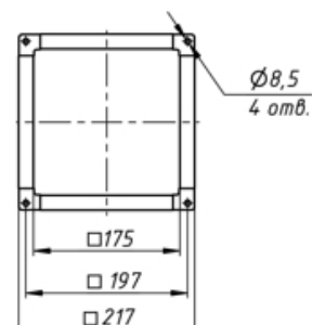
ВЫХОДНОЙ ФЛАНЕЦ
