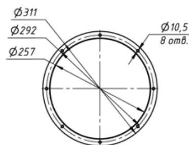
ВЫХОДНОЙ ФЛАНЕЦ
