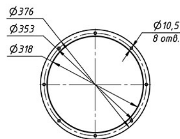
ВХОДНОЙ ФЛАНЕЦ
