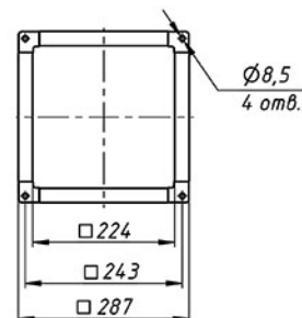
ВЫХОДНОЙ ФЛАНЕЦ
