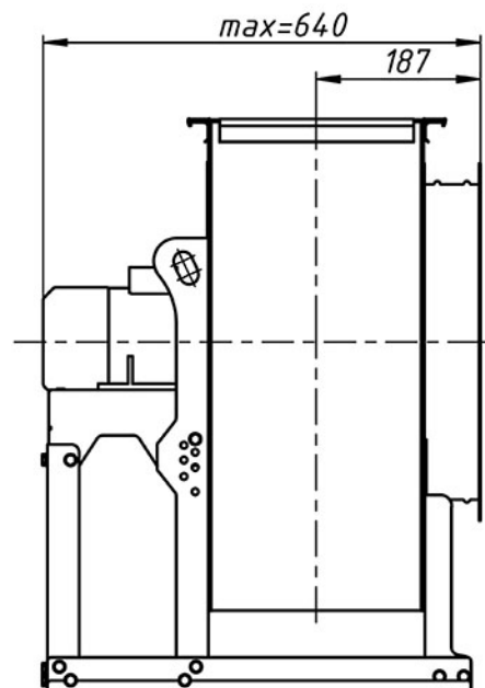
ВХОДНОЙ ФЛАНЕЦ
